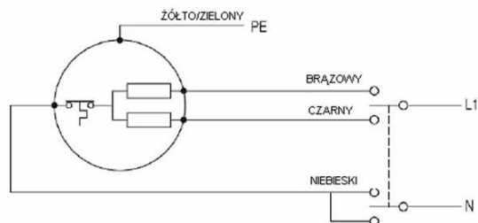
SCHEMAT POŁĄCZENIA SILNIKA DO PRZEŁĄCZNIKA WIELOBIEGUNOWEGO
